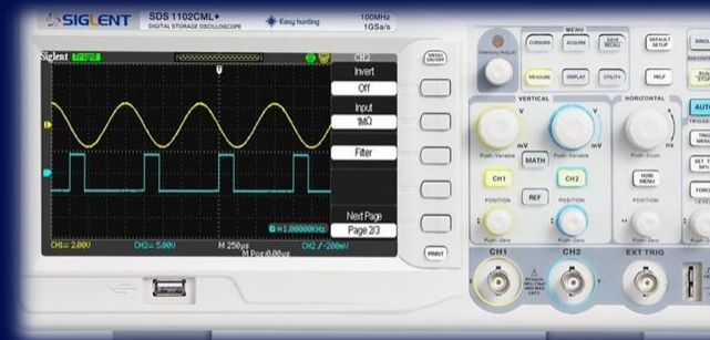
Siglent 1102 CML+
